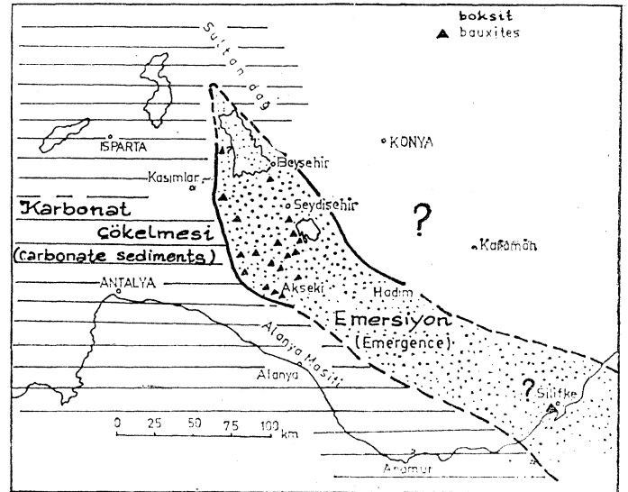
Şekil 11: Akseki-Seydişehir yöresinin Senomaniyen'deki paleoocoğrafik durumunu gösteren şematik harita.
