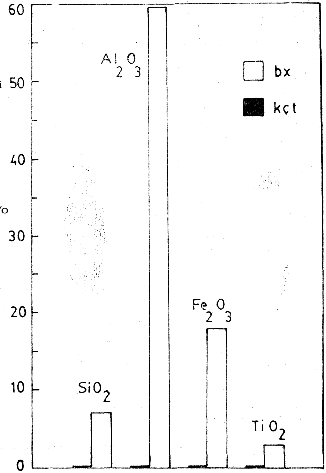
Sekil 2: Boksit ve kireçtaşlarında bazı oksit yüzdelerinin karşılaştırılması (bx: boksit, kçt: kireçtaş).
